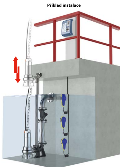
Příklad instalace
